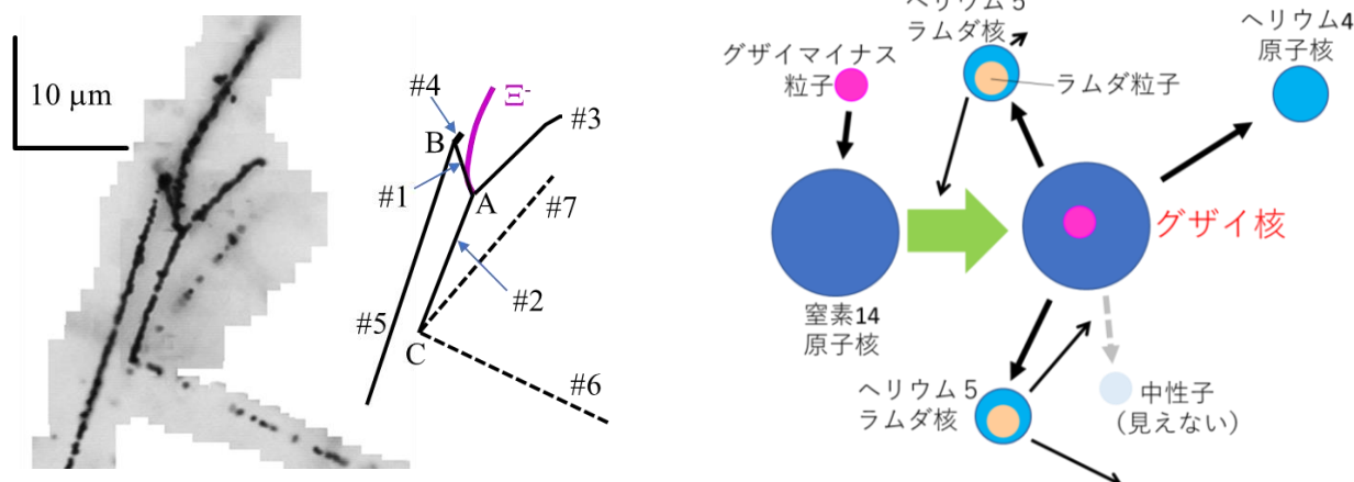
図 1. 写真乾板で観測された新たなグザイ核事象（イラワジ事象）の顕微鏡写真とそのイメージ図
