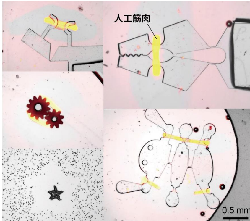
図 2. 人工筋肉の応用例 大きき数ミリメートルのシリコンゴム製の微小構造の周囲に、光照射により人工筋肉を形成させ、その構造を駆動させた。右上) マイクログリッパ：光照射後に人工筋肉（オレンジ色）が形成し、20 秒後にグリッパが閉じる。右下) 昆虫型デバイス：人工筋肉により左右に動く。左上) ロボットアーム型デバイス。左中) 微小歯車の組み立て。左下) 細胞サイズの微小ビーズの集積。
