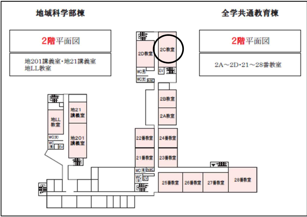
全学共通教育棟 2階 平面図
