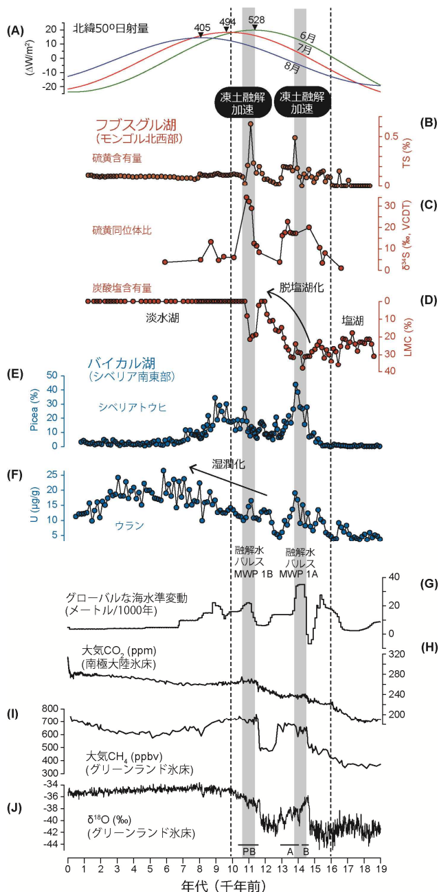
図2. 永久凍土融解の復元図。フブスグル湖の湖底堆積物中の硫黄含有量の増加と硫黄同位体比の正異常が13,700年前と11,000年前に見られ、永久凍土の急激な融解が生じたことが明らかとなった。また、同様にして、バイカル湖周辺でも土壌水分やシベリアトウヒの増加が認められた。これらの時期は、南極氷床コアから復元された大気CO 2 濃度、グリーンランド氷床コアの大気CH 4 濃度、珊瑚による海水準が急激に増加した時期と対応することが明らかとなった。図中のBはベーリング期、Aはアレレード期、PBはプレボレアル期を表す。MWP1Aは融解水パルス1A、MWP1Bは融解水パルス1Bを表し、大陸氷床の融解に伴い世界中の海水準が年間40mmの速度で急激に上昇した。
